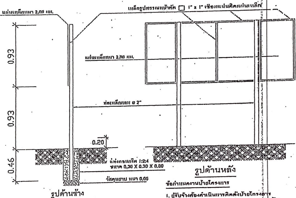
แบบป้ายโครงการ ยাত্রาส่วน 1:30
